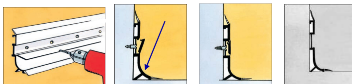
4442093 - Plinthe de 80mm G2
