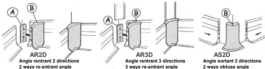
Pièces de finition rigides à fixations mécaniques cachées uniquement
